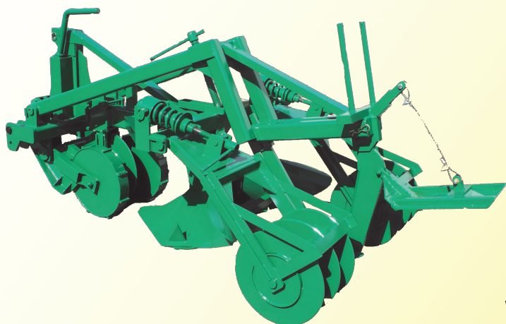
LPŻ-75 z pogłębiaczem i bez pogłębiacza
